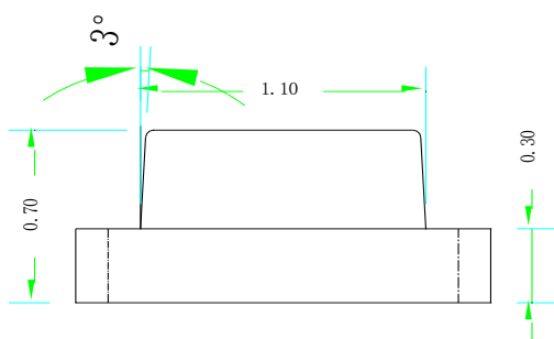
侧面视图
