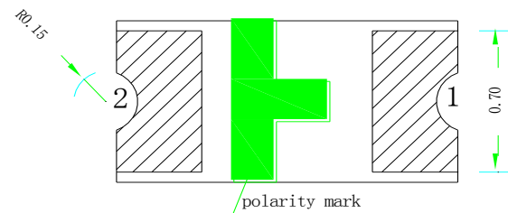
背面视图
