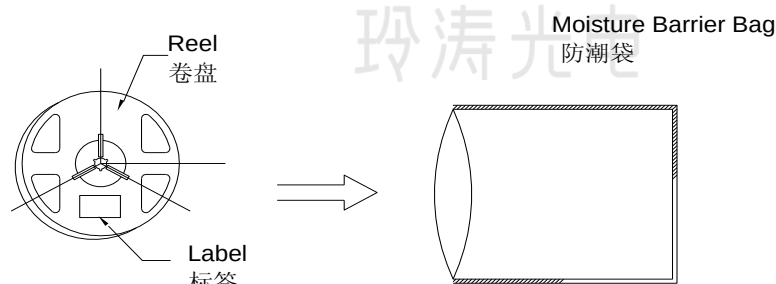
Fig 2-4 Moisture Resistant Packing Process 防潮包装过程
