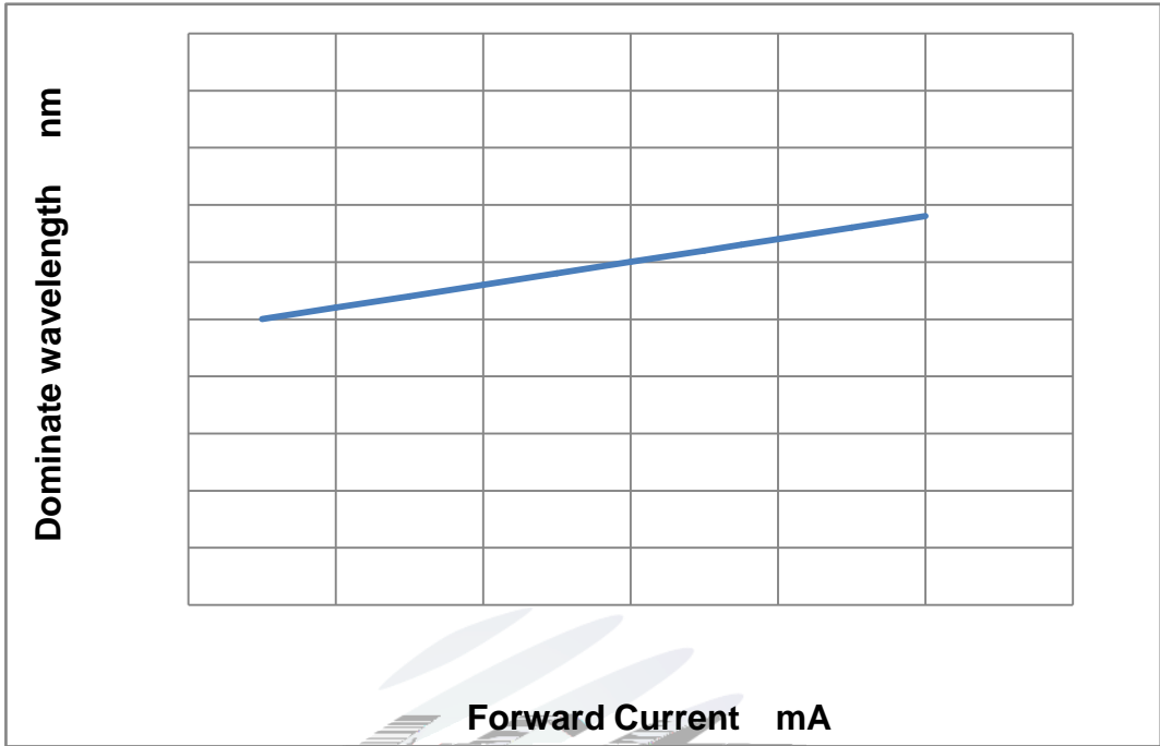
Fig. 1-13 Forward current vs. Dominate wavelength 正向电流与中心波长特性曲线 (Ts=25°C)
